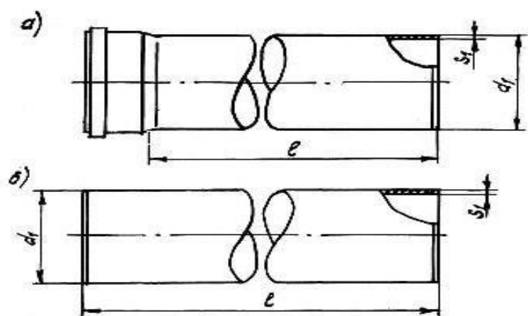
Рисунок 1. Конструкция и размеры труб
