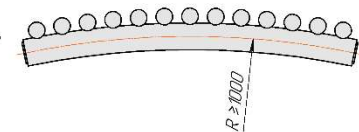
Гармония А 20-1нп R наружн., изготавливается без встроенного термоклапана
