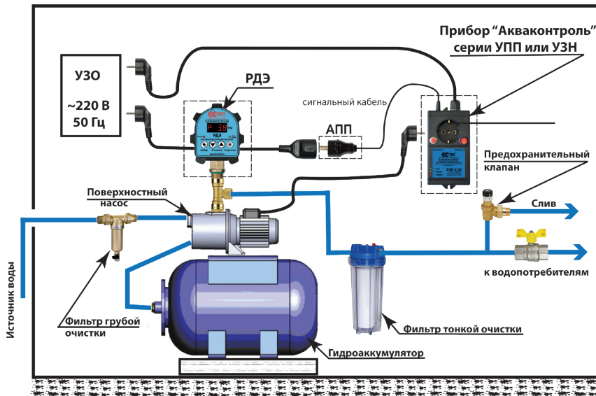
Пример 4. Подключение РДЭ для управления однофазным насосом мощностью P1 более 1,5 кВт, или трехфазным погружным насосом.
