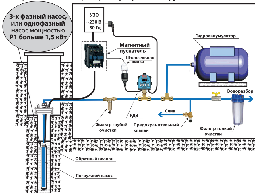
Пример 4. Подключение РДЭ для управления однофазным насосом мощностью P1 более 1,5 кВт, или трехфазным погружным насосом.
