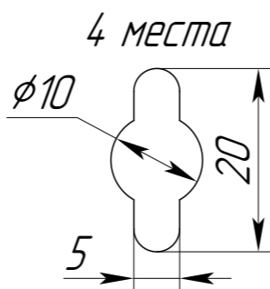
А (увеличено)
