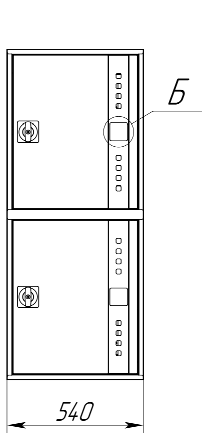
Вид спереди
