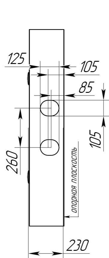
Вид справа
