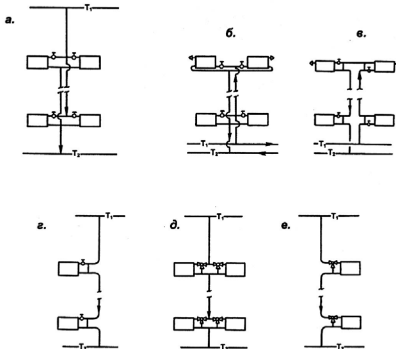
Рис. 2.2 Схемы вертикальных стояков систем водяного отопления: а, б – двухтрубные; в, г, д, е – однотрубные
