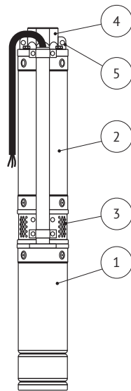
Рисунок 1 - Устройство агрегата
