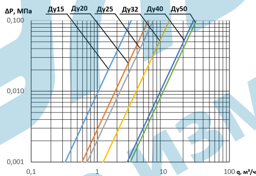
ПРИЛОЖЕНИЕ 2 Диаграмма потери давления
