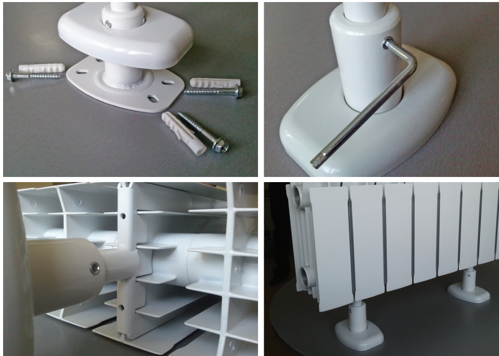
Рис.13 Порядок установки опор
