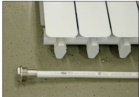
Рис.19 Удлинитель с ввинченным отрезком трубы
